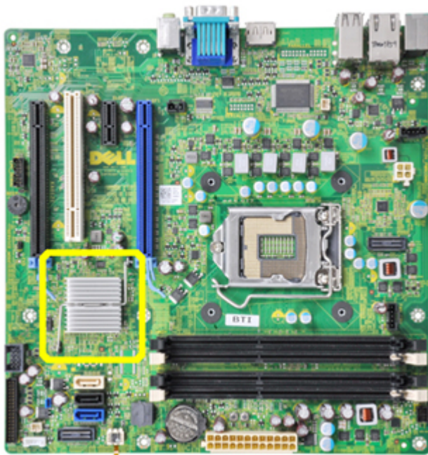
Figura 1. Scheda di sistema di una versione precedente rispetto alla scheda di sistema fornita con il dissipatore di calore
